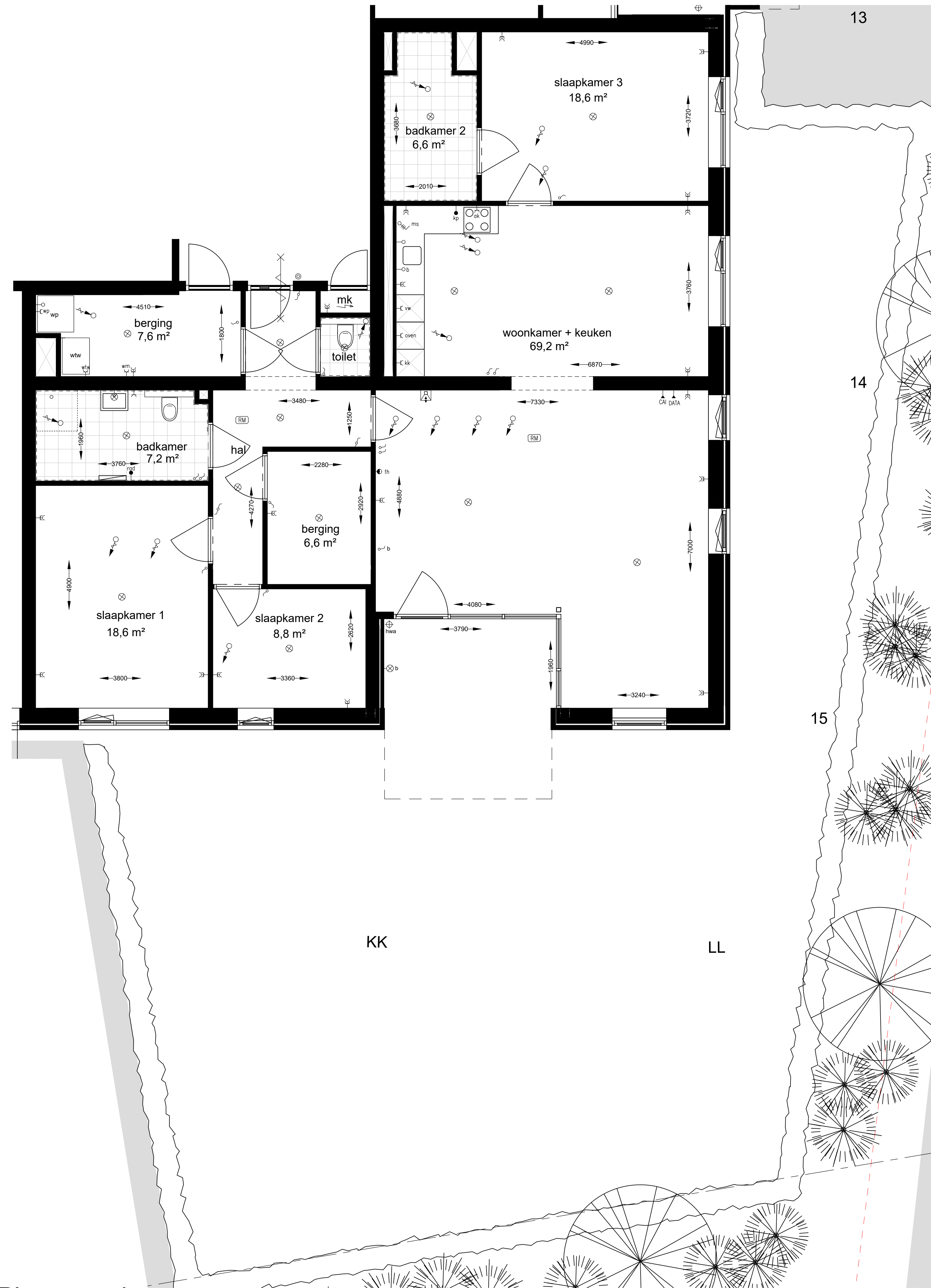
Plattegrond 1:50
