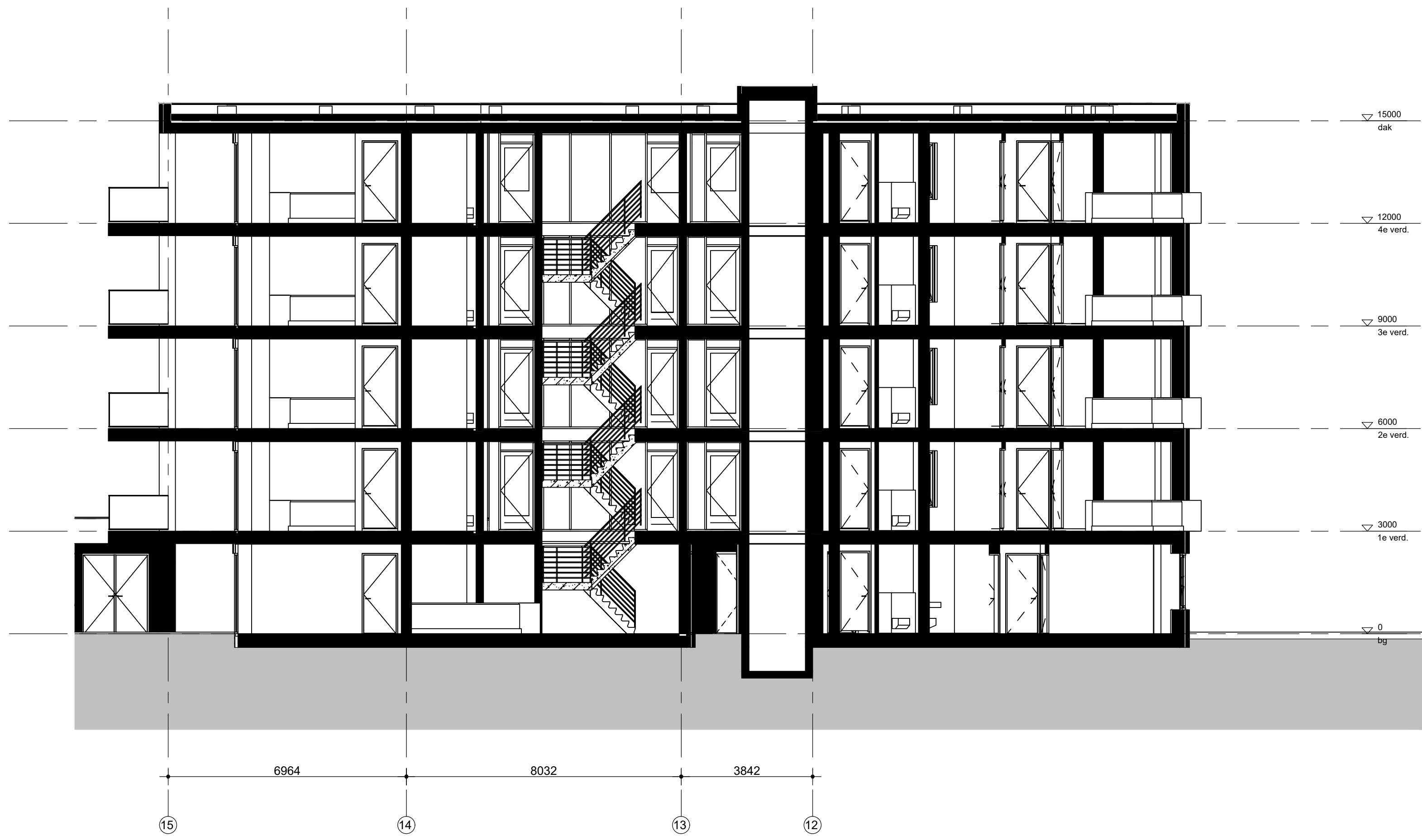
Langsdoorsnede 1:100
