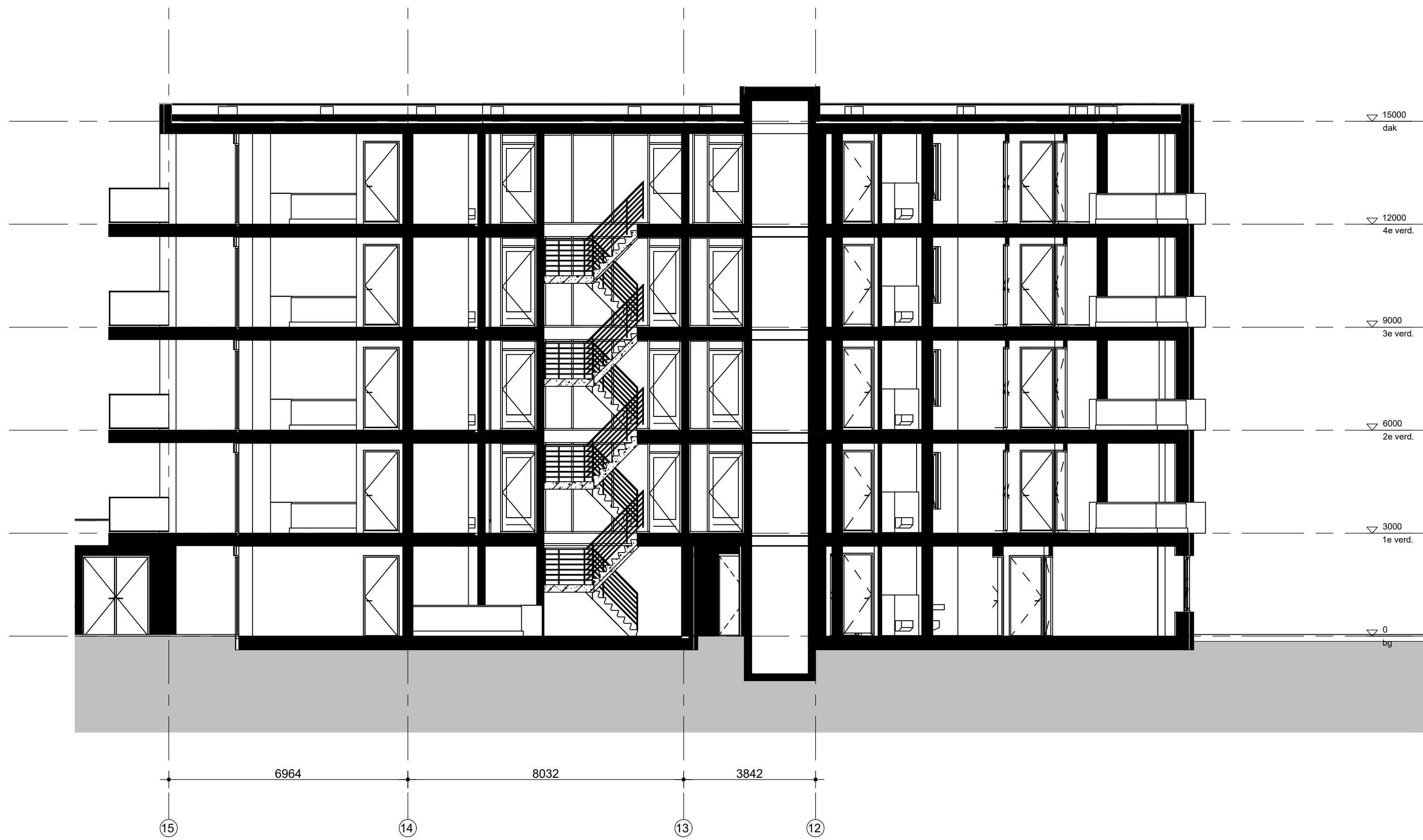
Langsdoorsnede 1:100
